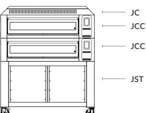
COMP - 2ST SUPPORTO CON GUIDE PORTATEGLIE E RUOTE STAND WITH TRAYHOLDER SLIDES AND CASTORS
