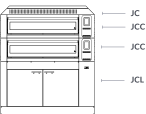
COMP - 2CL CELLA DI LIEVITAZIONE CON RUOTE PROVING CHAMBER WITH CASTORS
