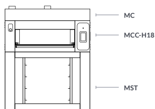
COMP1 M18-ST SUPPORTO CON GUIDE PORTATEGLIE STAND WITH TRAYHOLDER SLIDES
