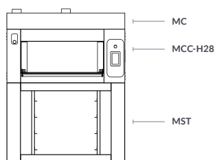
COMP1 M28-ST SUPPORTO CON GUIDE PORTATEGLIE STAND WITH TRAYHOLDER SLIDES
